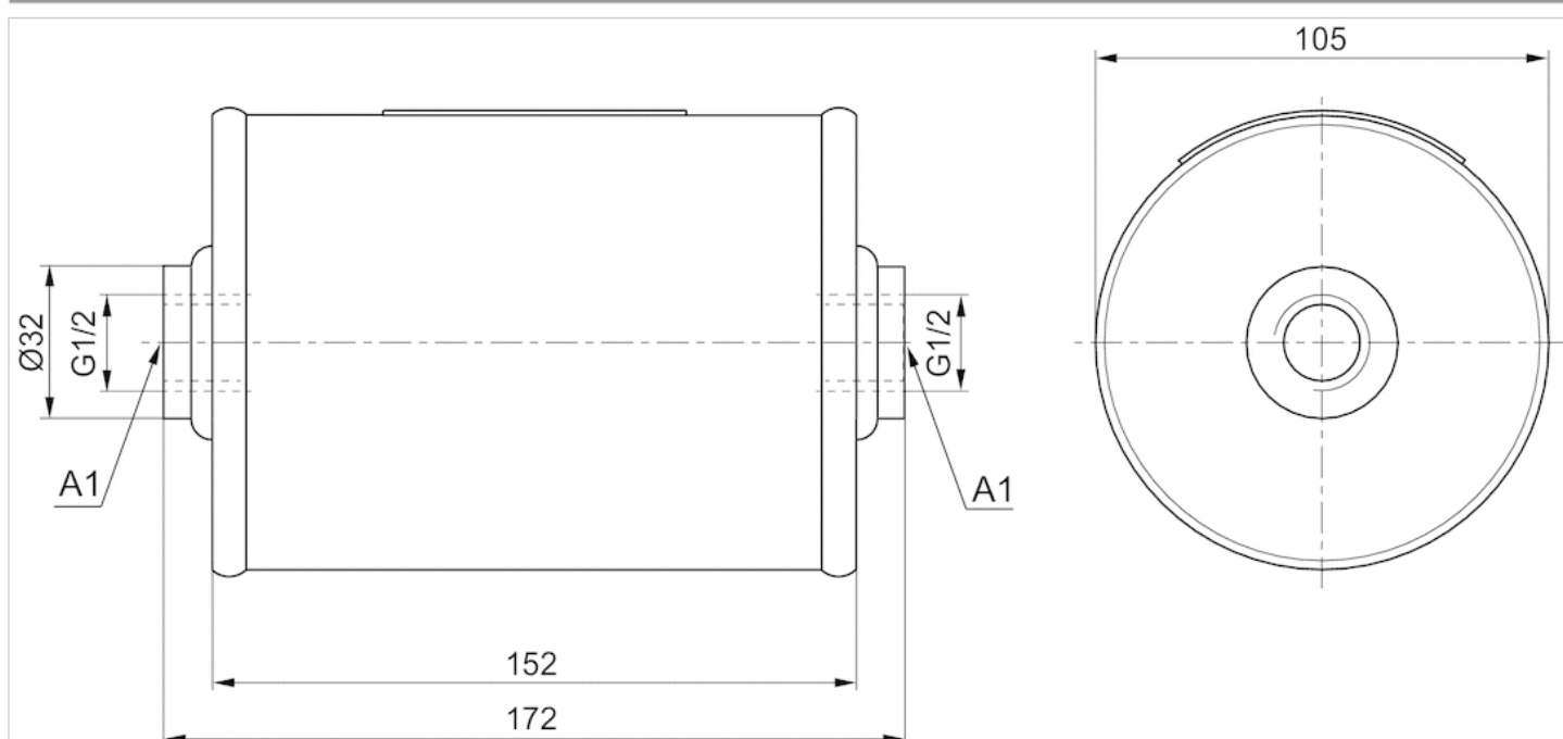
Abmessungen Fig. 1
