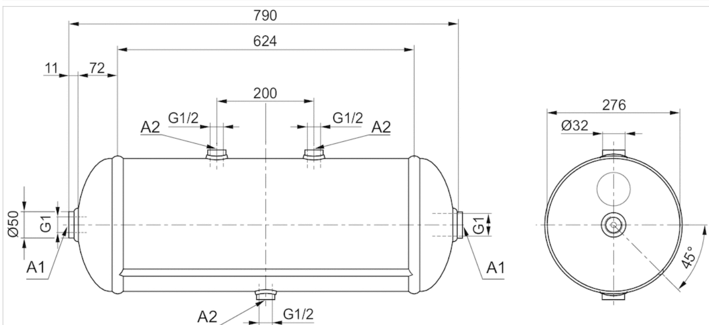
Abmessungen Fig. 6
