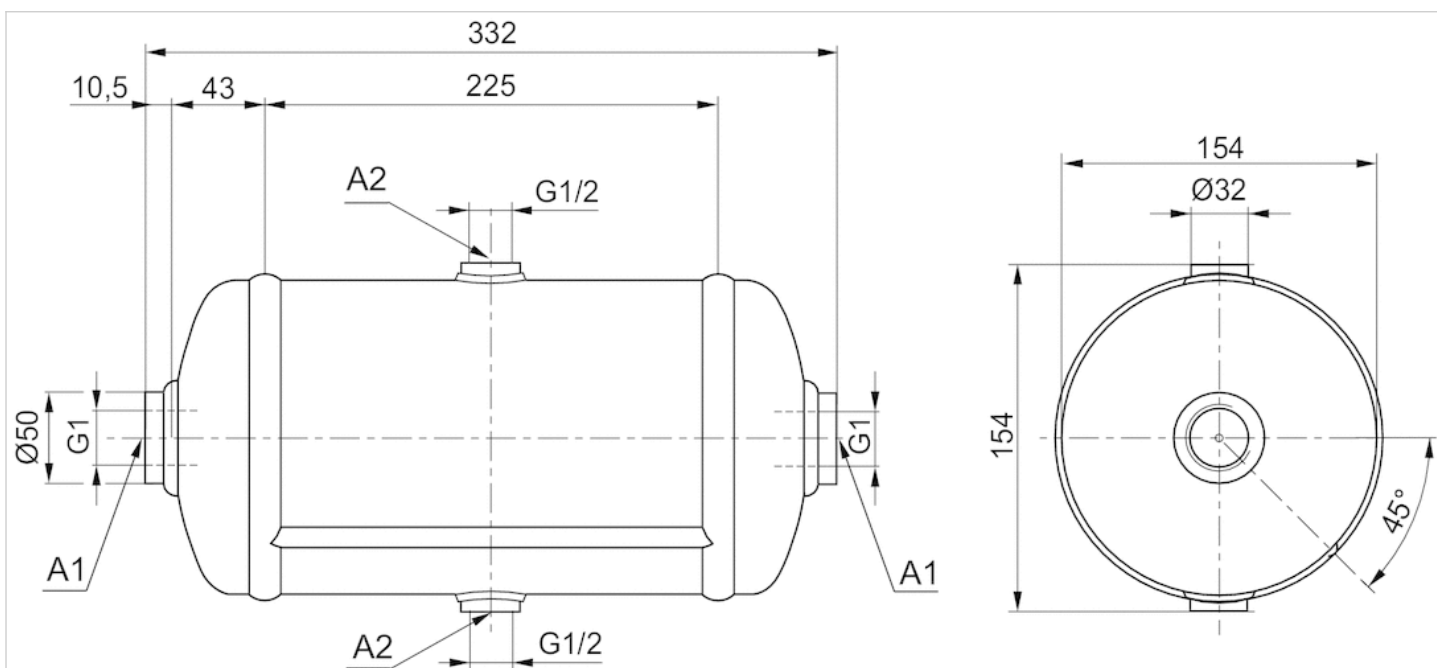
Abmessungen Fig. 3
