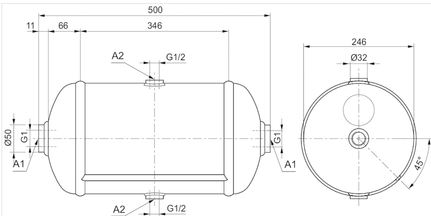
Abmessungen Fig. 5
