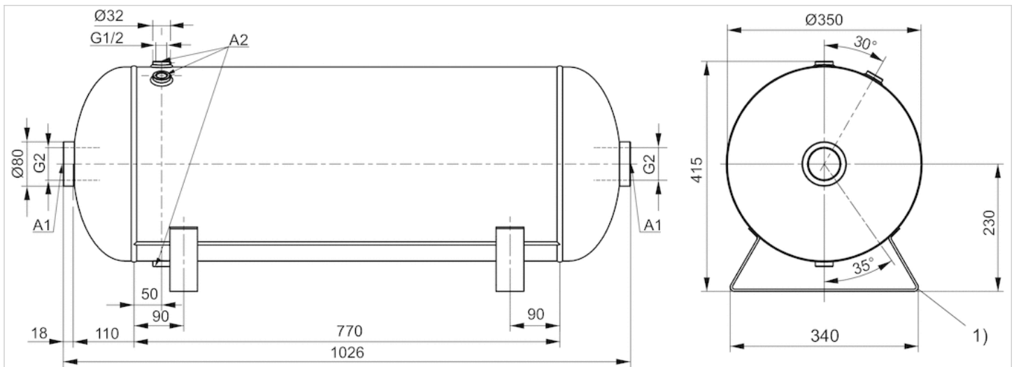
Abmessungen Fig. 7
