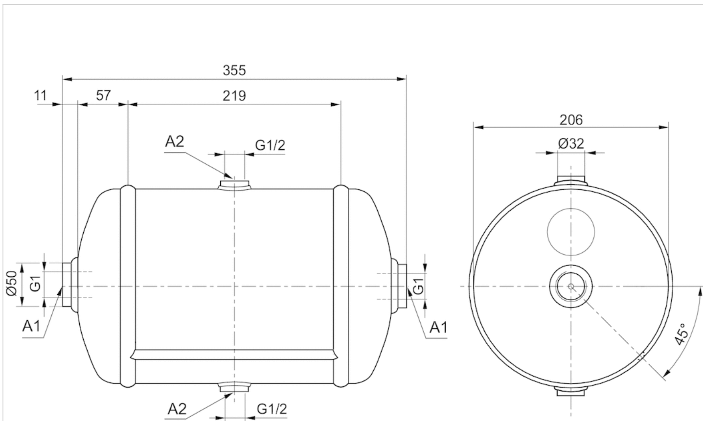
Abmessungen Fig. 4
