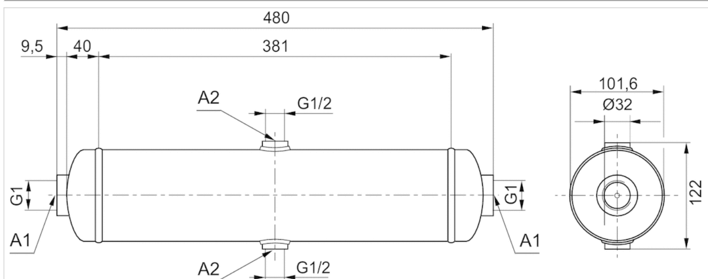
Abmessungen Fig. 2
